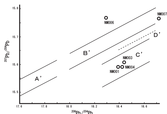
図6 鉛同位体比の関係図（B式図）
